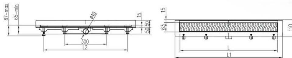
ROZMĚRY ŽLABU
